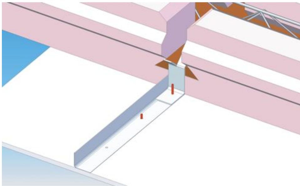
Detalj podkonstrukcije za montažu gips kartonskih ploča na strop. Ankerna ploča se ugrađuje u toku be
